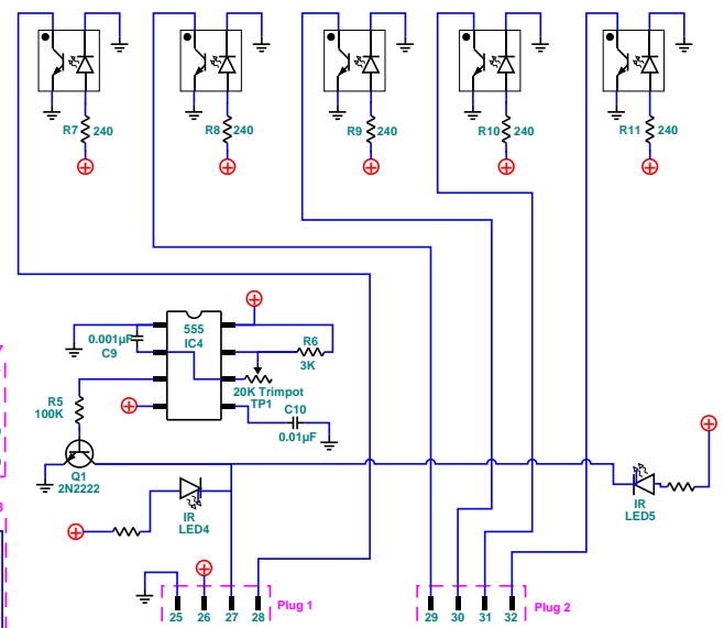
Edge Sensor Board PCB
